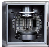
ラウンダーメータ外観 紫外線フェードメータ試験槽 図2 染色堅ろう度試験に使用する機器
