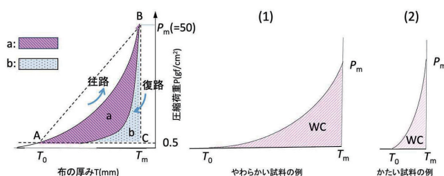
図1 圧縮測定のプロットイメージ
