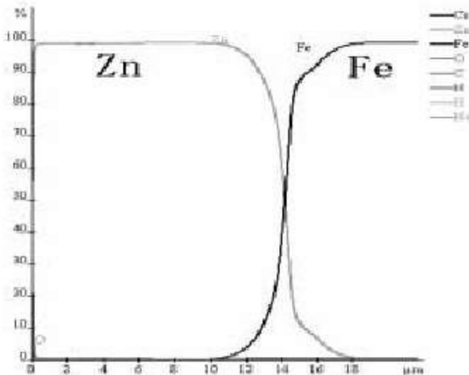
▲亜鉛メッキした鋼板の測定事例
